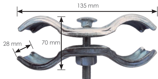
Bride renforcée
