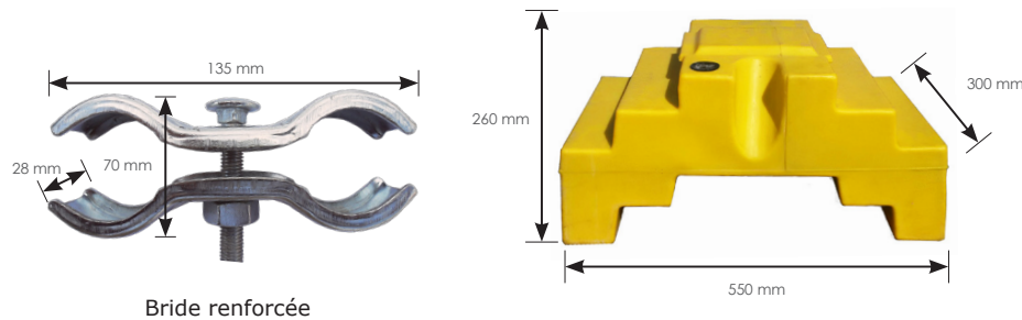
Bride renforcée
